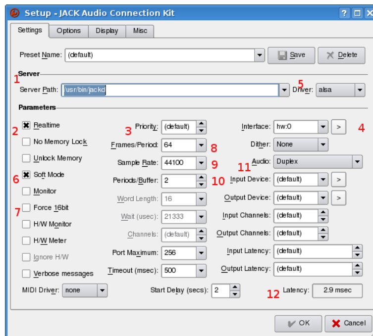
Figuur 3.2: Setup
